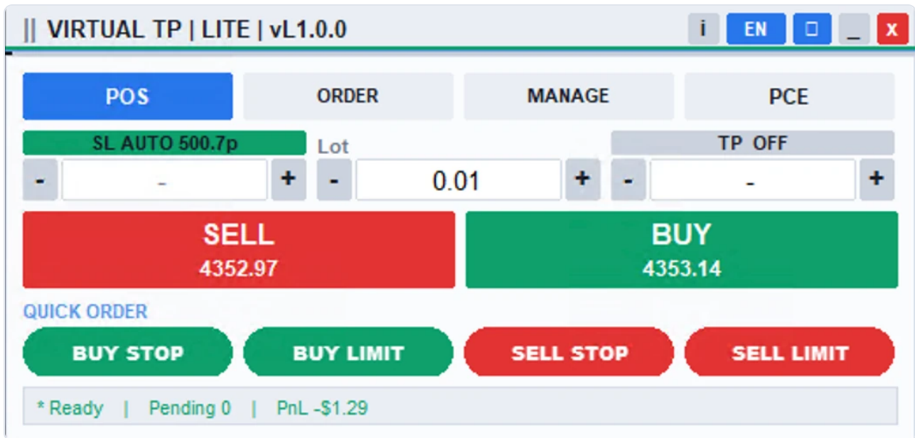
Gambar 6 — Tab POS — kotak SL, kolom Lot, kotak TP, tombol SELL dan BUY, lalu baris Quick Order di bagian bawah.
